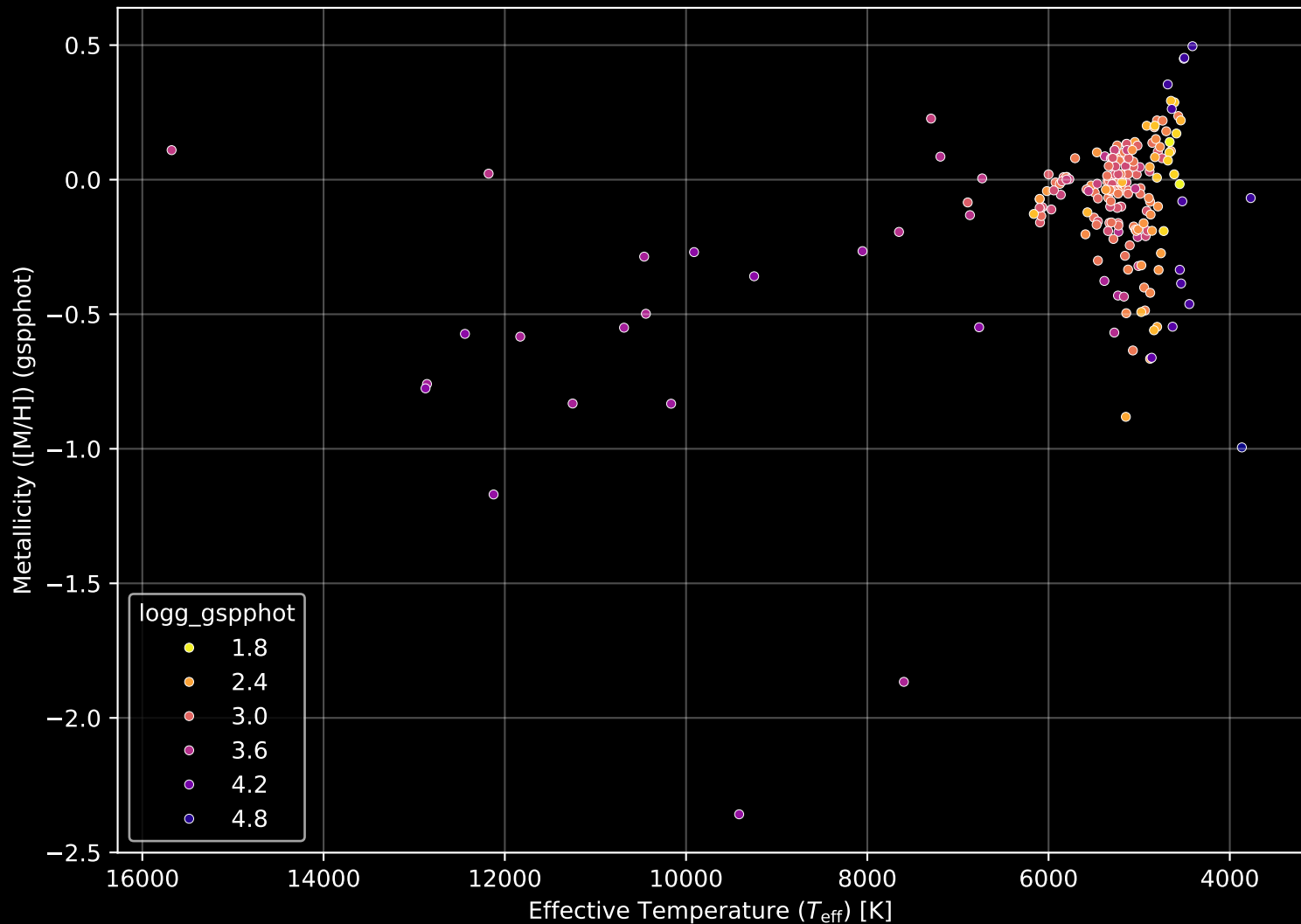
APOGEE DR17 Field: [158-04] Stellar Population Parameters (n= 208)
